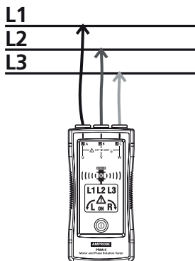
Figura 1: Tabla de indicación de fase (también impresa en la parte posterior del medidor PRM-6)
