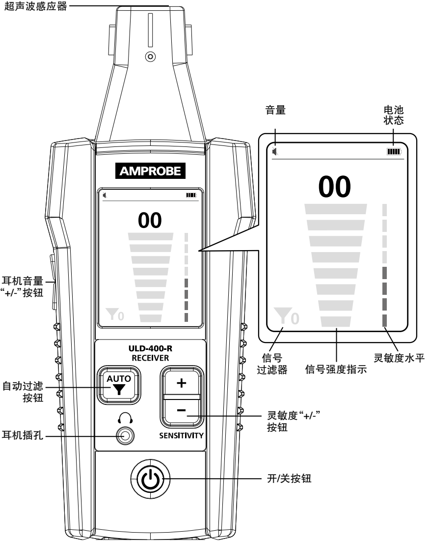
图3.2: ULD-400-R接收器
