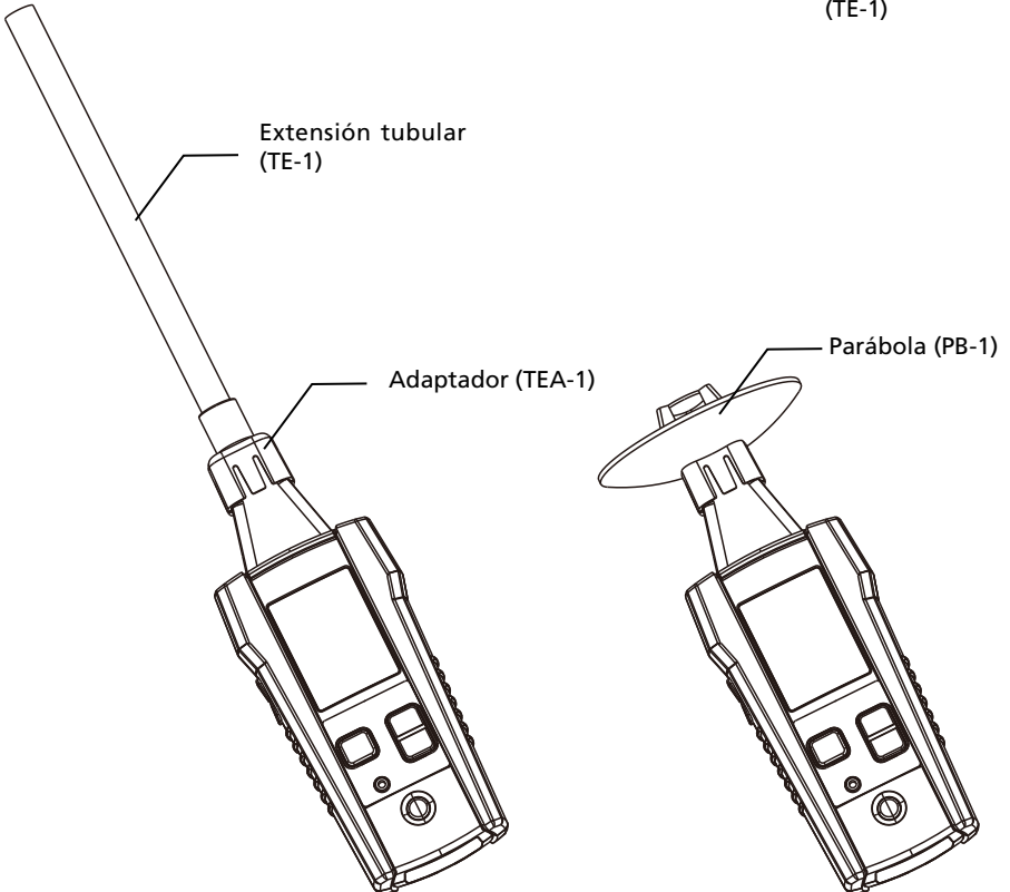
Figura 3.4: Accesorios ULD-400
