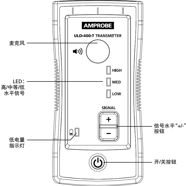
图3.3: ULD-400-T发送器
